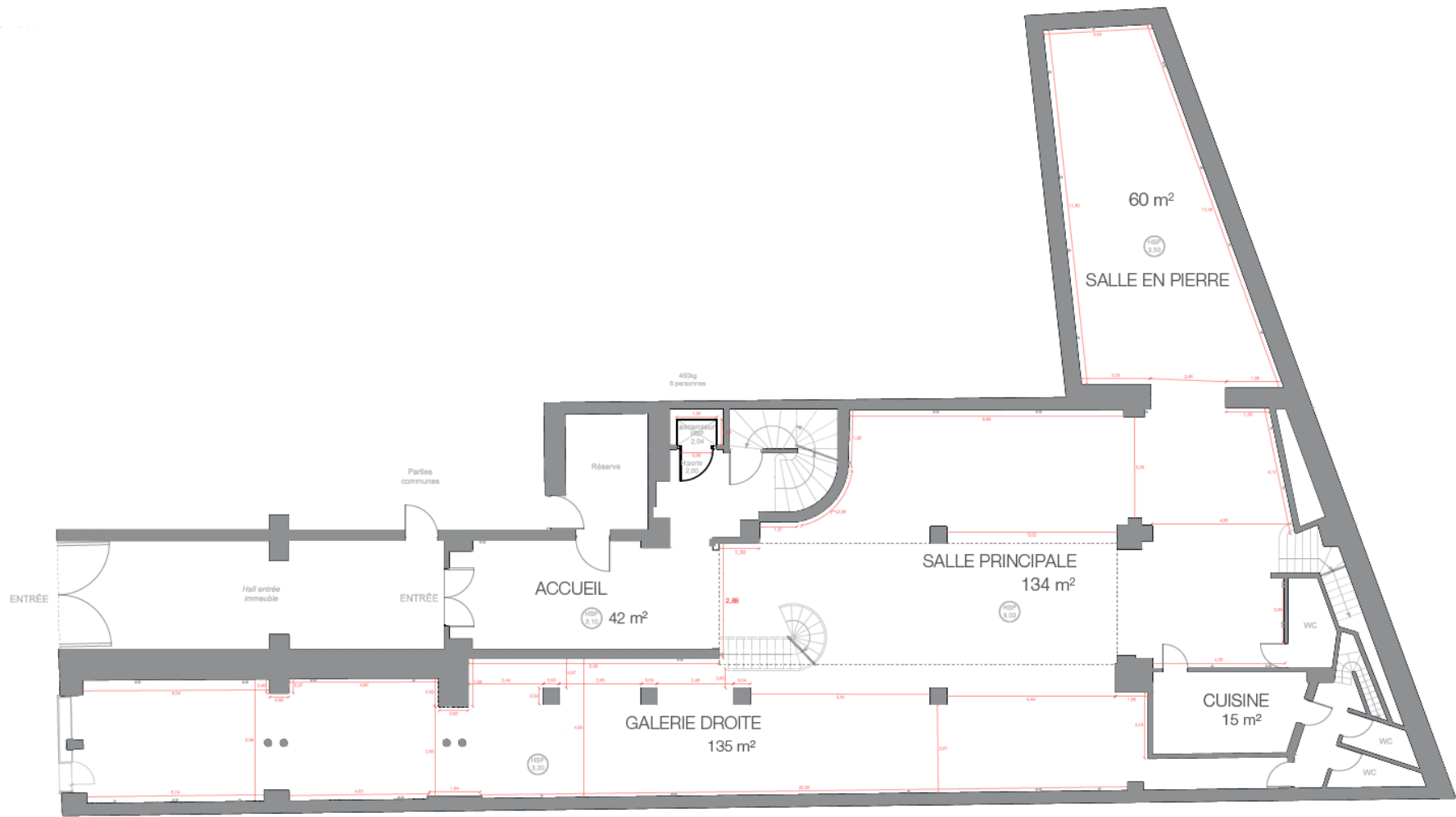
PLAN REZ-DE-CHAUSSÉE
